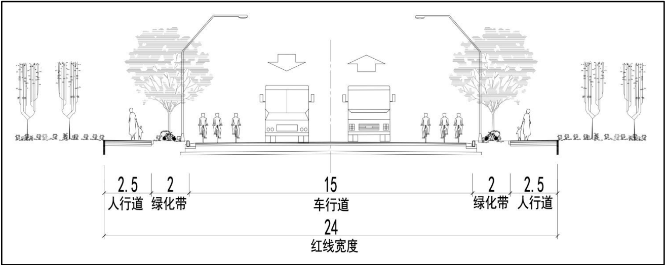
道路标准横断面图
