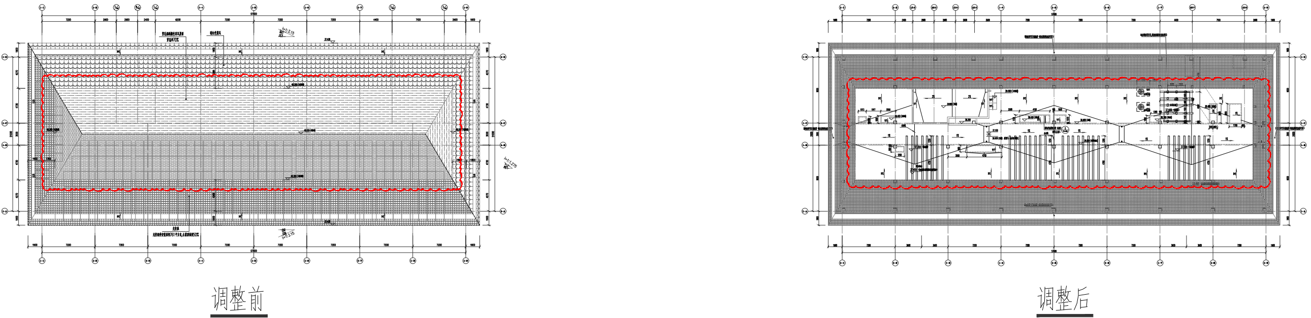
附图3：1#教学实训大楼屋顶穿孔板装饰构架取消。
